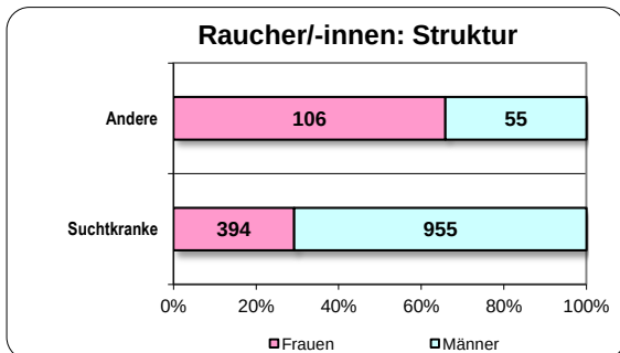
Abb. 16: Raucher/-innen: Struktur
