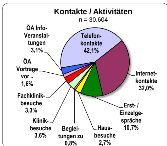
Abb.5: Kontakte / Aktivitäten
