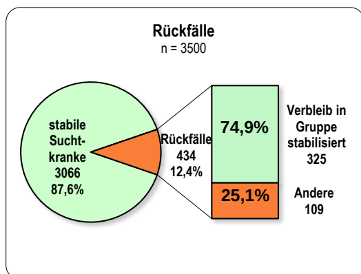
Abb. 21: Rückfälle
